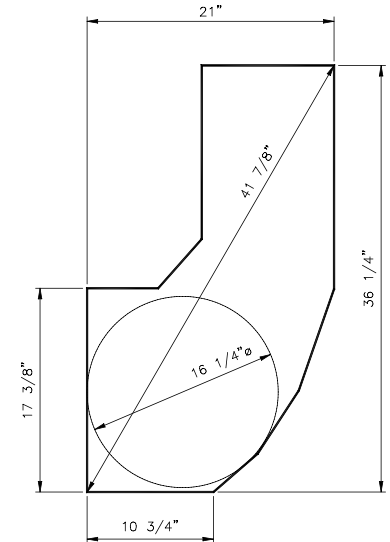
Goulotte de la déchiqueteuse de 65"
