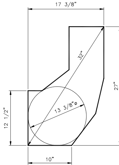
Goulotte de la déchiqueteuse de 55"
